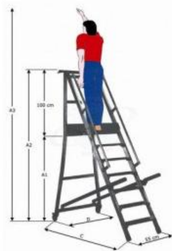
Leiter mit Arbeitsplattform h55_56
